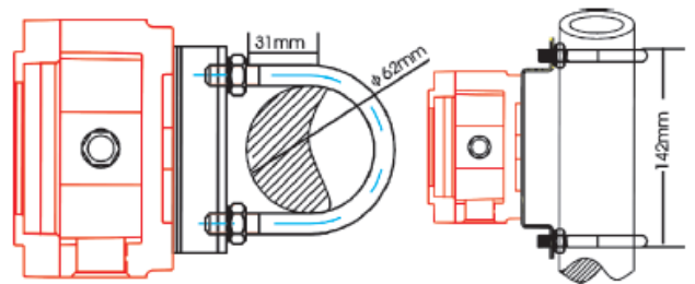
管道支架安装图
