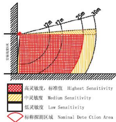
探测器水平向下45° 视角图
