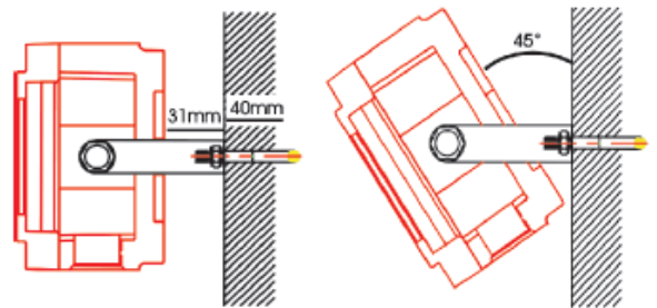
墙壁安装侧视图
